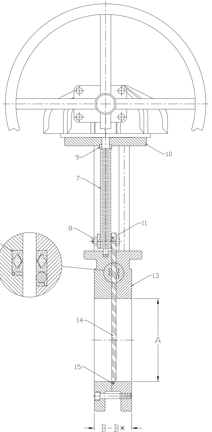
SECTION A-A
