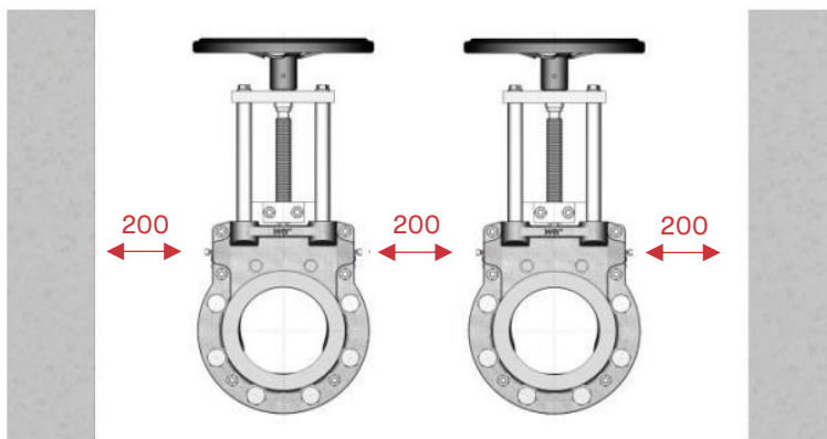
Abbildung 2: Einbaustelle
