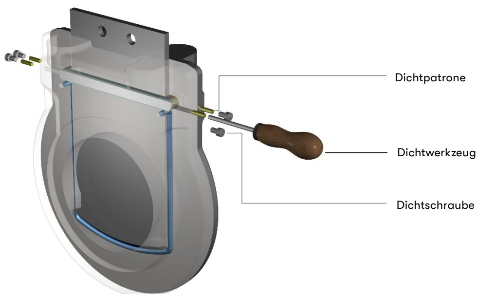
Abbildung 7: Nachdichten
