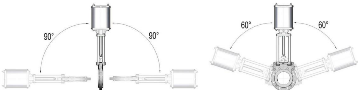
Abbildung 3: Einbaulage
