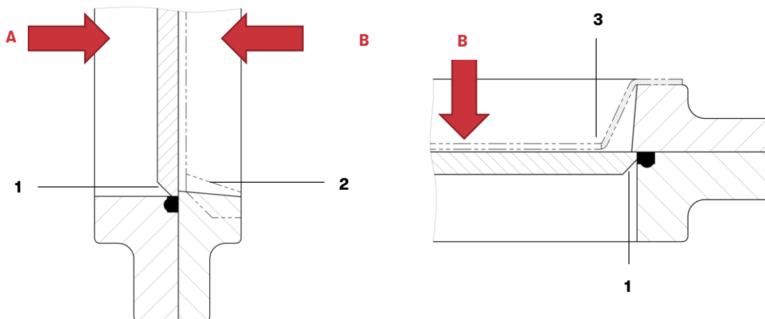
Abbildung 4: Druckrichtung
