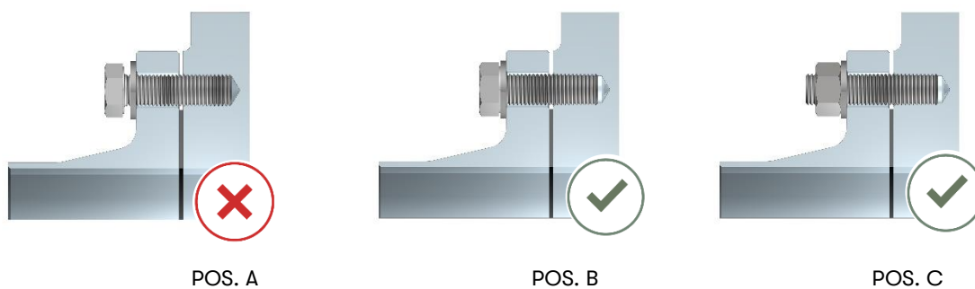
Abbildung 5: Montage Flansch-Schrauben
