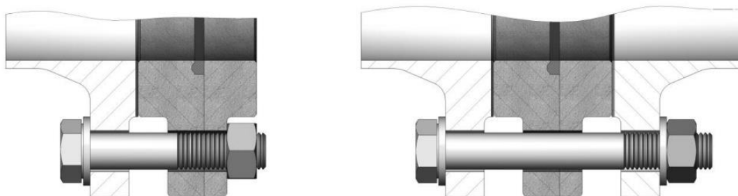
Einbau als Endschieber
