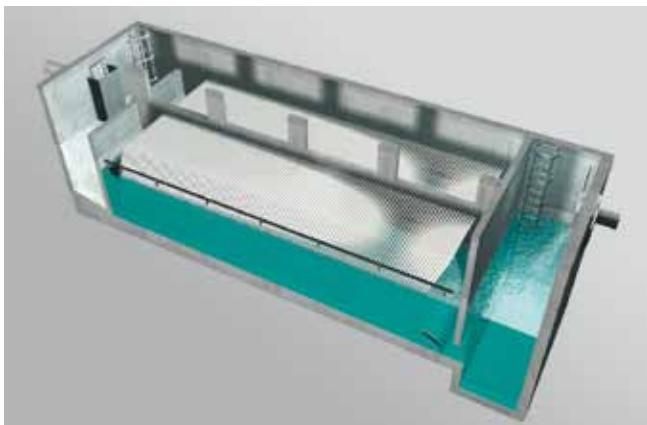
HydroM.E.S.I Partikelabscheider Partikelabscheider für Regen- und Mischwasser, Strassenwasserbehandlungsanlagen
