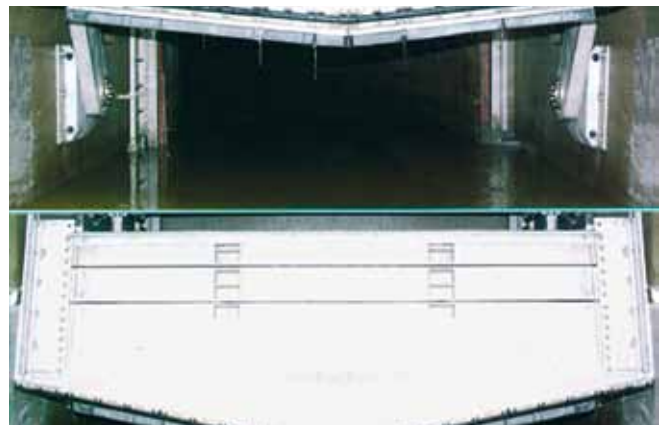
HydroGuard Spül- und Stauschutz zur kompletten Bewirtschaftung von Kanalnetzen
